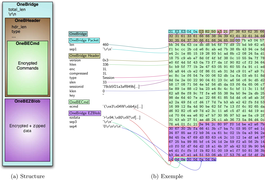
Fig. 9. Paquet chiffré
