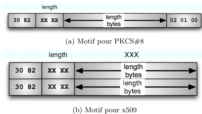
Fig. 2. Motifs à rechercher en mémoire
