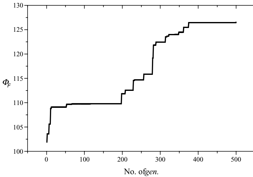
(b) \Phi_F vs. gen.
