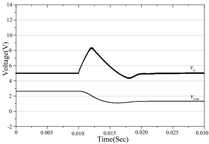
(a) v_o and v_{con} .
