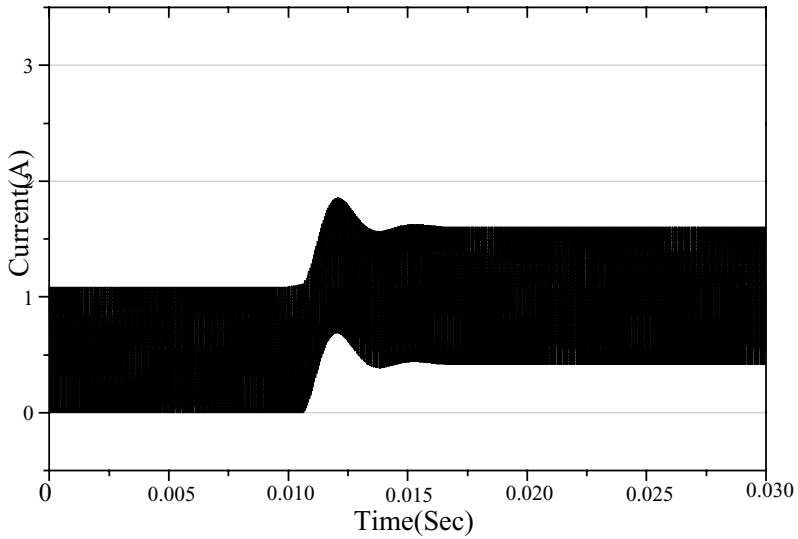
(b) i_L
