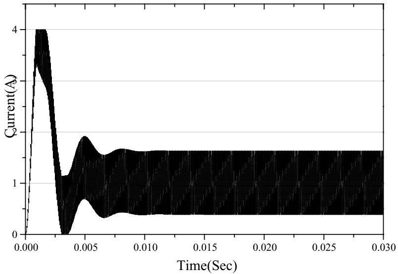
(b) i_L .
