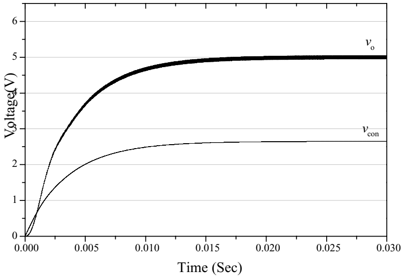
(a) v_o and v_{con} .
