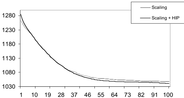
(d) Mean fitness evolution with fitness2
