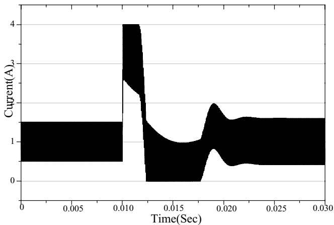
(b) i_L .
