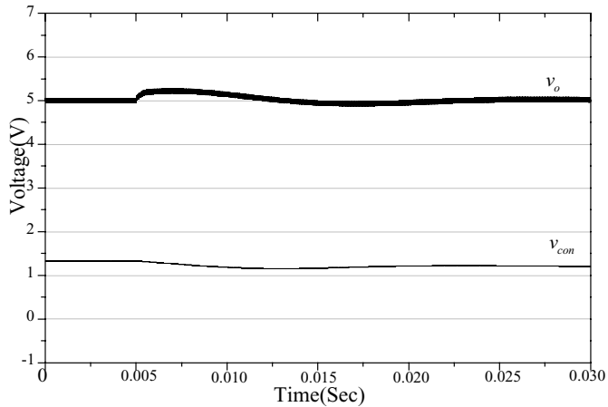
(a) v_o and v_{con} .
