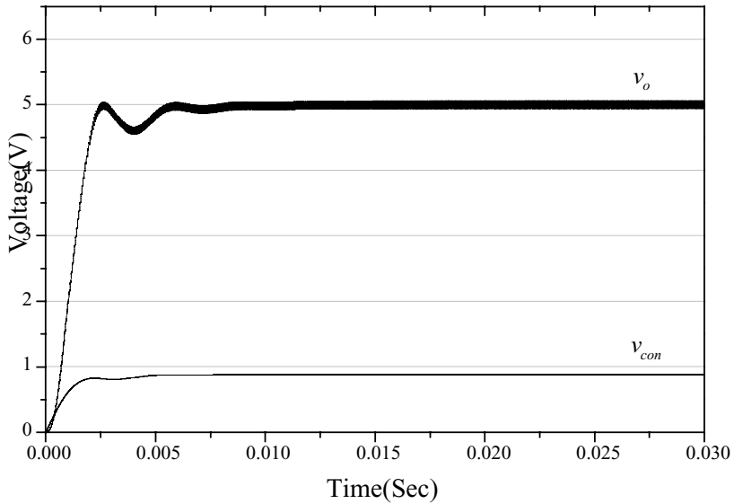
(a) v_o and v_{con} .
