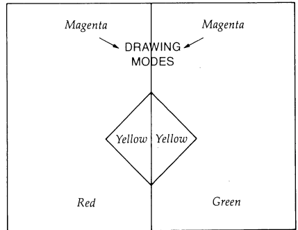
Mode 2-Jam 1
