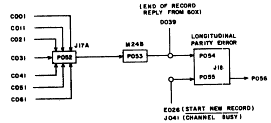
LONGITUDINAL PARITY CHECKER
