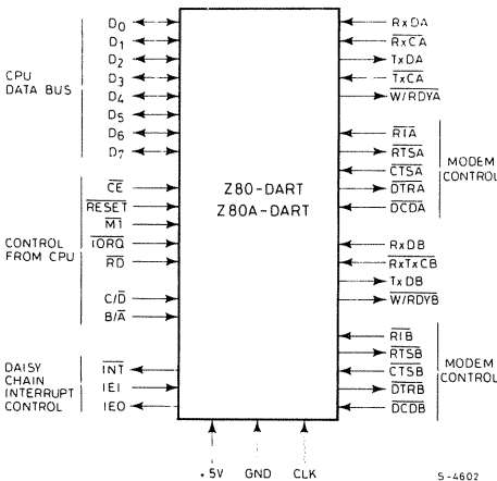
Fig. 1 - PIN FUNCTION
