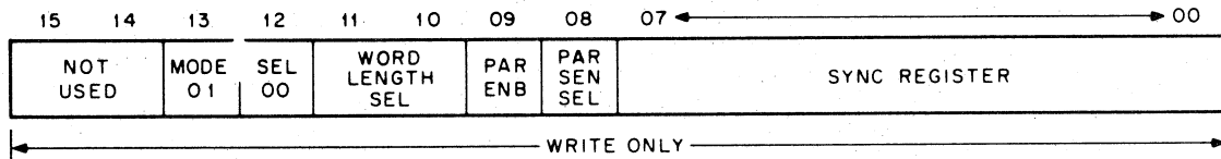
Figure 3-3 Parameter Status Register (PARCSR)
