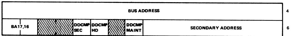
CNTL I FORMAT
