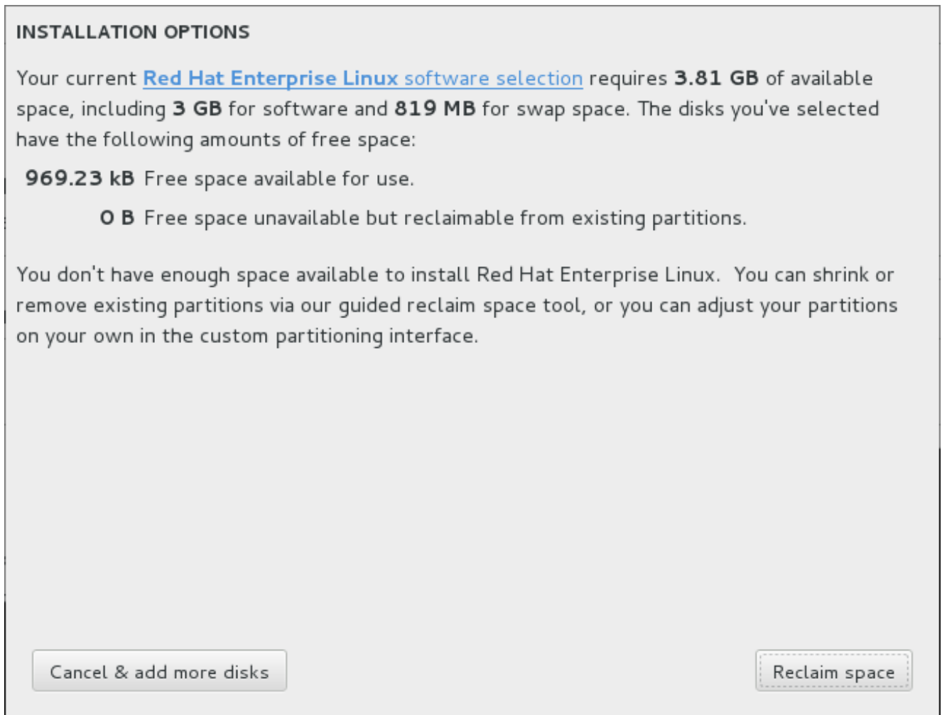
Figure 6.19. Boîte de dialogue des options d'installation avec option de récupération d'espace
