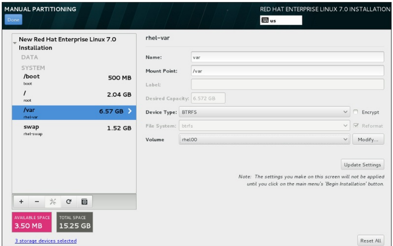
Figure 6.30. Configurer un sous-volume Btrfs
