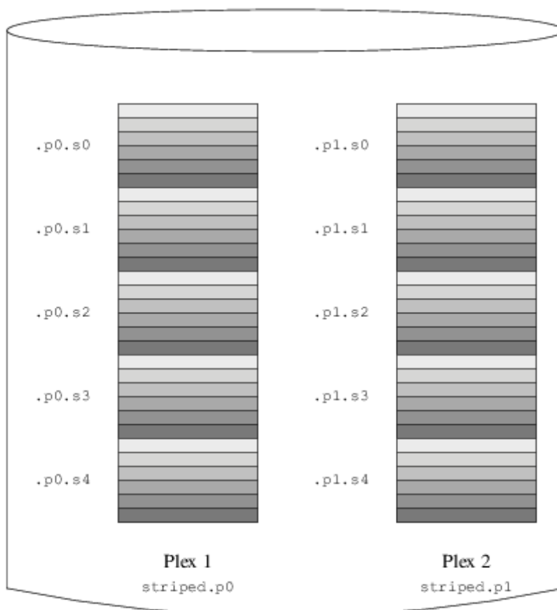
Figure 21.7. Un volume Vinum en mode miroir segmenté
