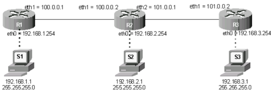
Topologie de travail
