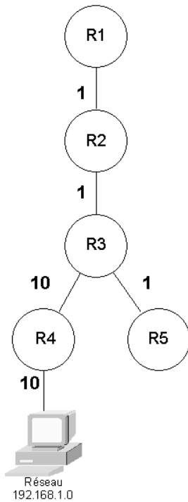
Topologie vue de R1
