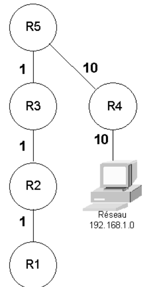
Topologie vue de R5
