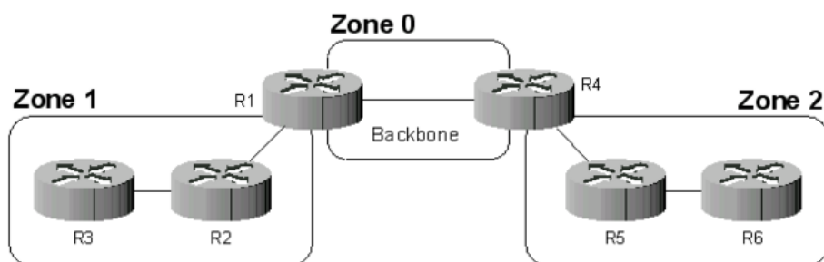
Réseau découpé en trois zones
