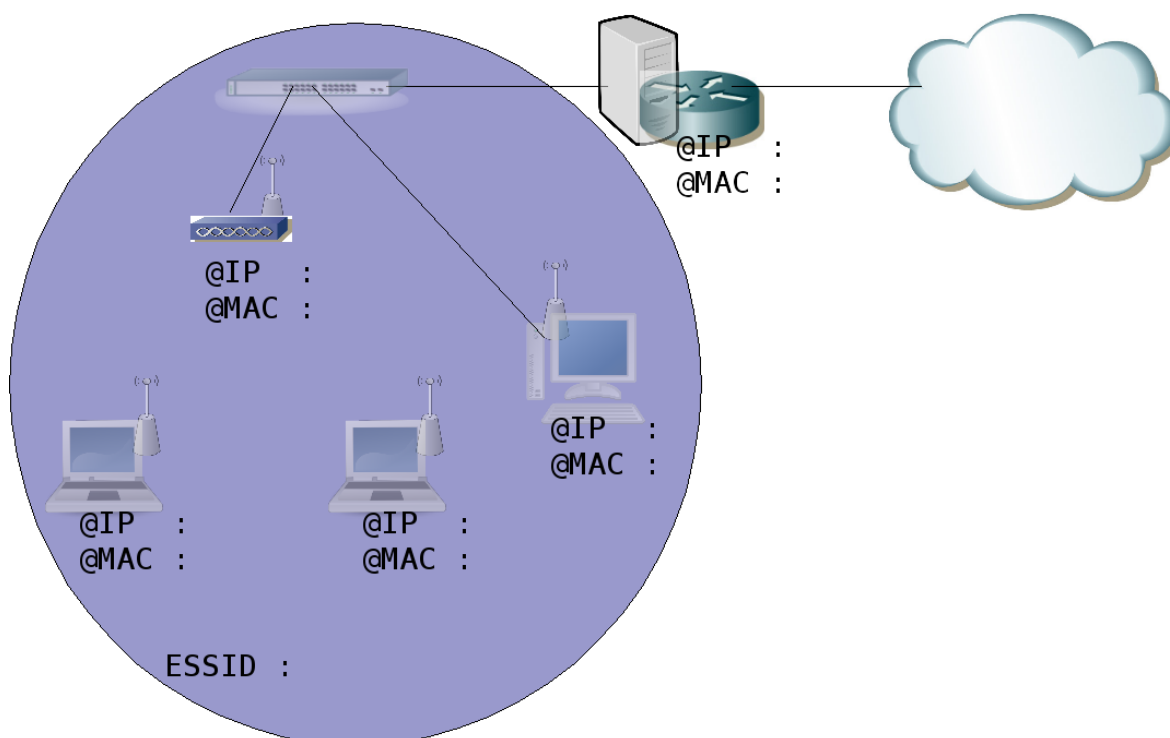
Schéma type d'infrastructure réseau sans-fil - vue complète 10
