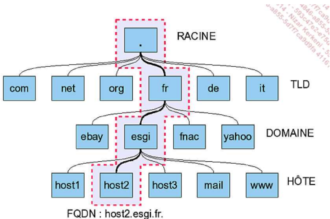
Représentation d'une arborescence DNS
