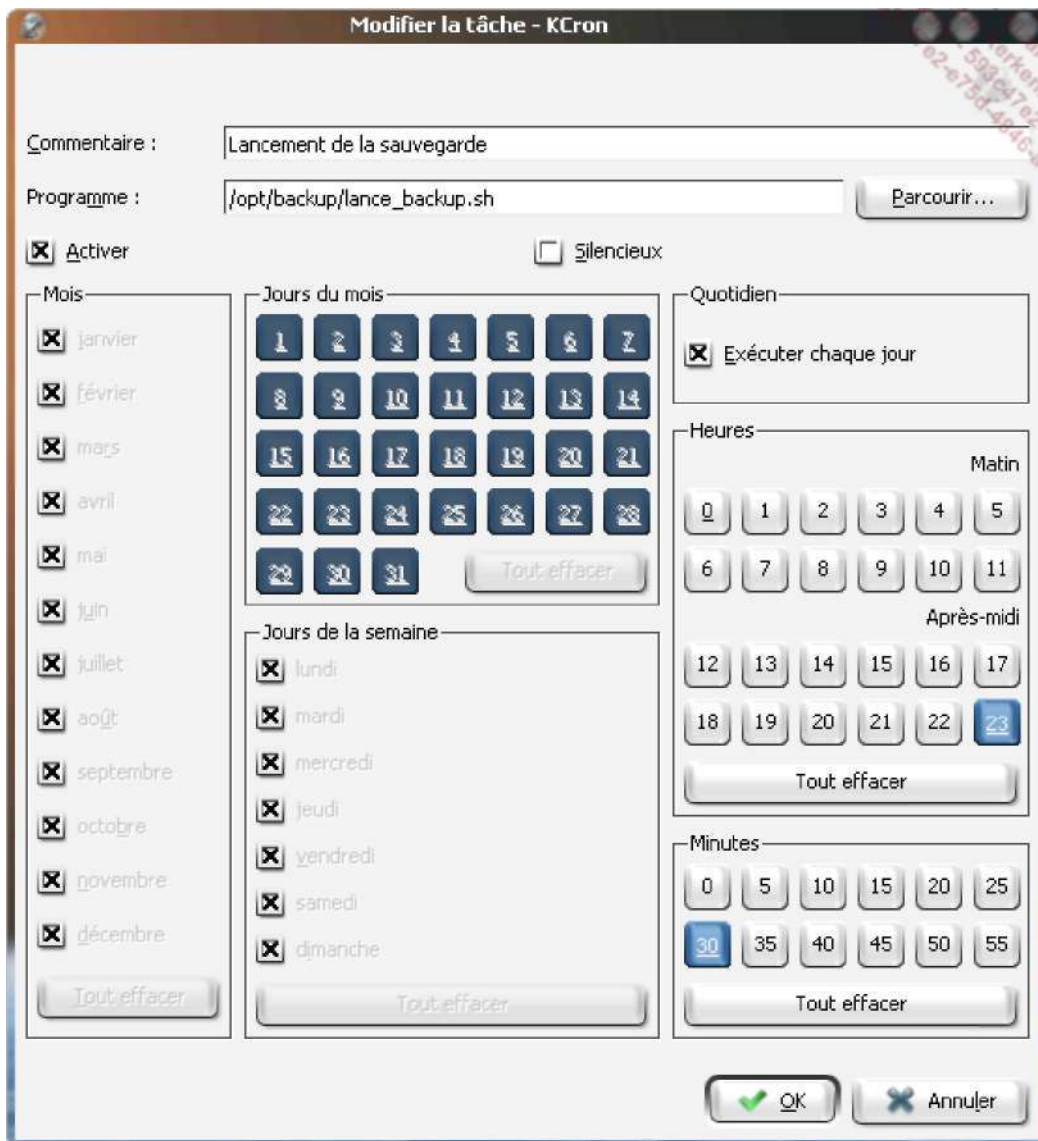
L'outil kron sous KDE
