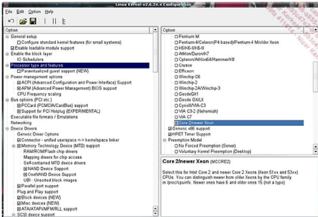
Les options de compilation via xconfig
