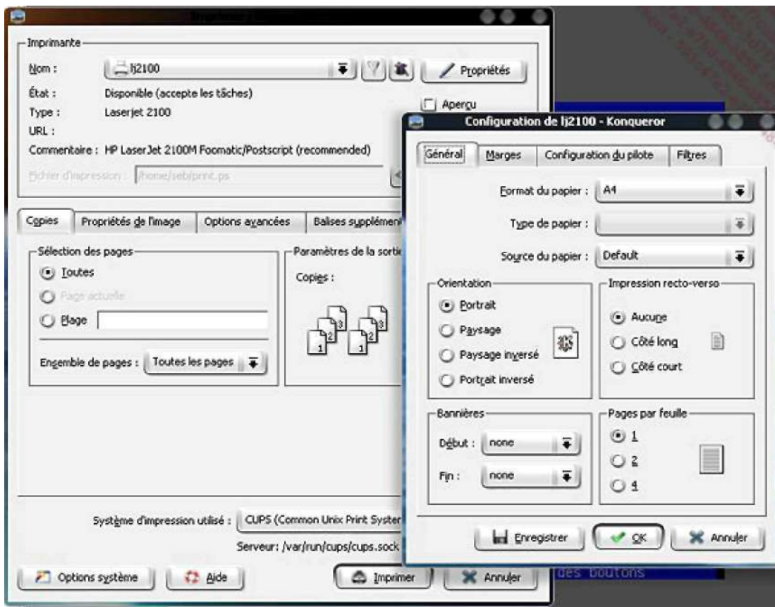
Boîtes de dialogue d'impression sous KDE
